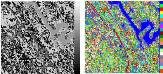
Output sampel A dg PCA
