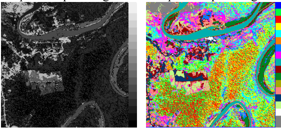
Output sampel B dg PCA
