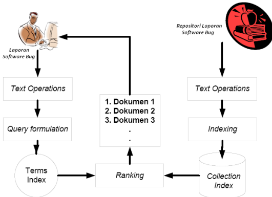
Gambar 4. Arsitektur Sistem
