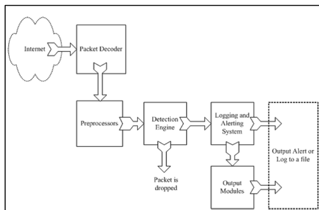
Gambar 1. Komponen Snort
