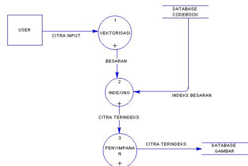
Gambar 2. Proses Penyimpanan data
