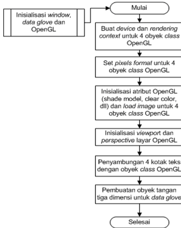
Gambar 3: Diagram alir inisialisasi
