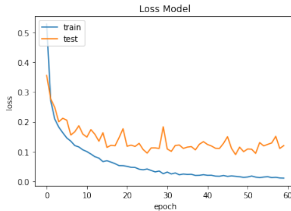
Gambar 5. Grafik Hasil Loss Pemodelan CNN
