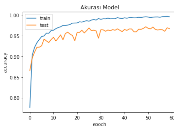
Gambar 4. Grafik Hasil Akurasi Pemodelan CNN.
